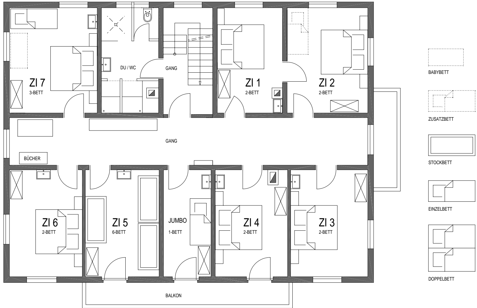
1.Obergeschoss 22 SCHLAFPLÄTZE
